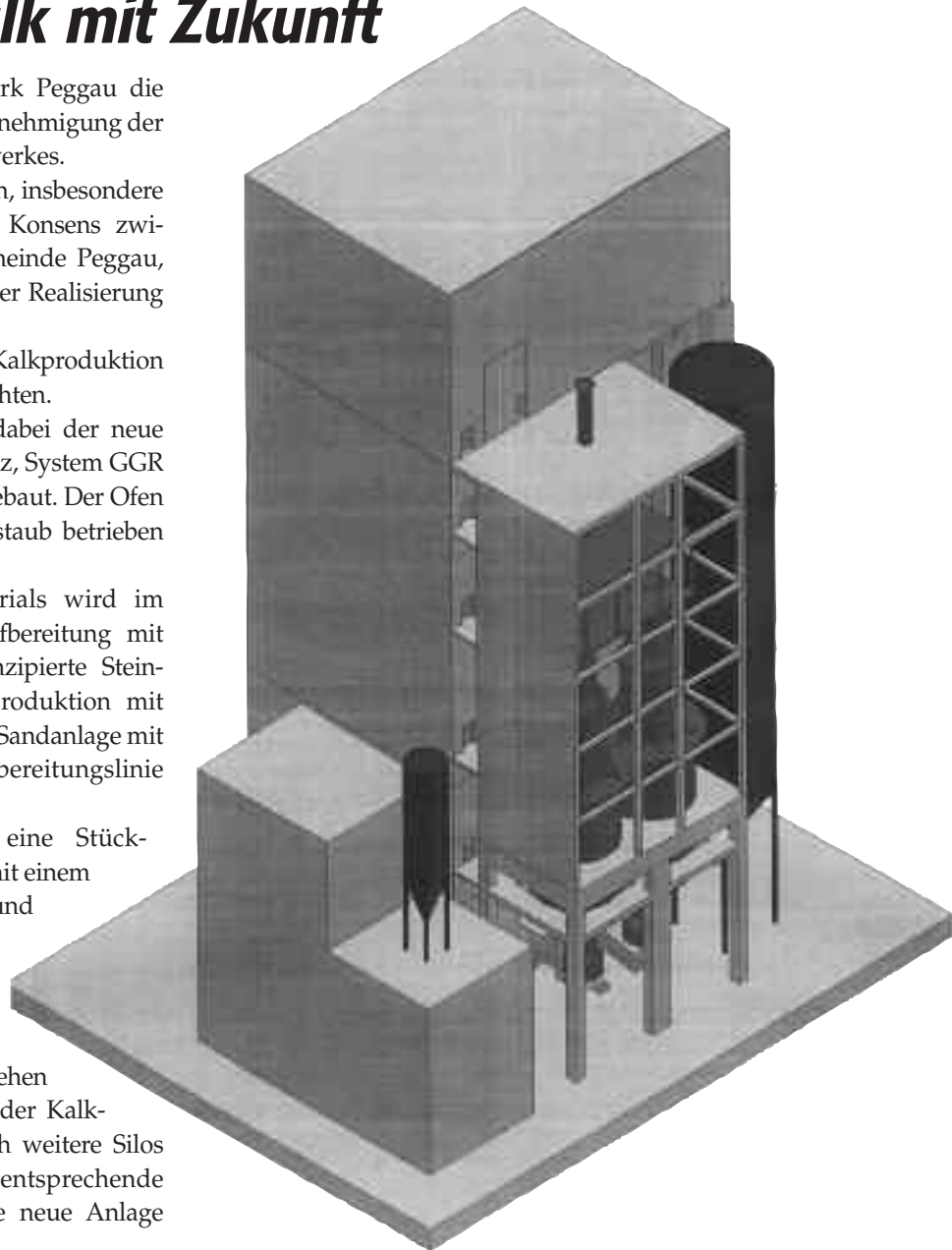
Dreidimensionale Darstellung des neuen Kalkofens.
